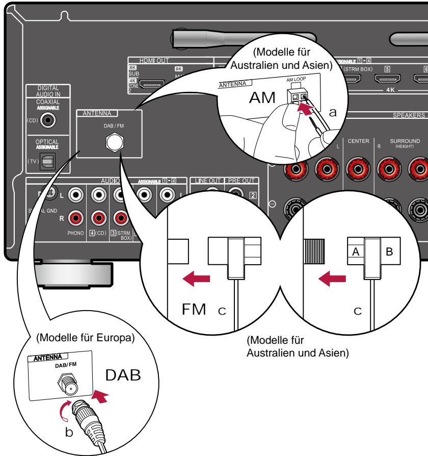
a AM-Rahmenantenne, b DAB/FM-Antenne, c FM-Zimmerantenne
