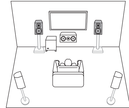
5.1-Kanal (Bi-Amping (Front)) ( → p26 )
