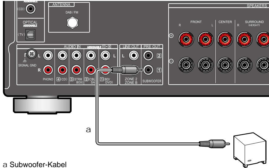
a Subwoofer-Kabel
